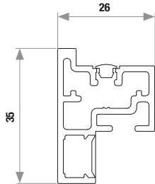
Perfil 3000 mm. frontal Lumix
